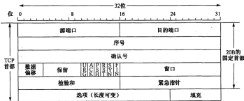
题 47-b 图 TCP 段头结构
