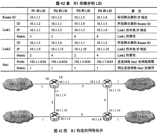
题 42 图 R1 构造的网络拓扑
